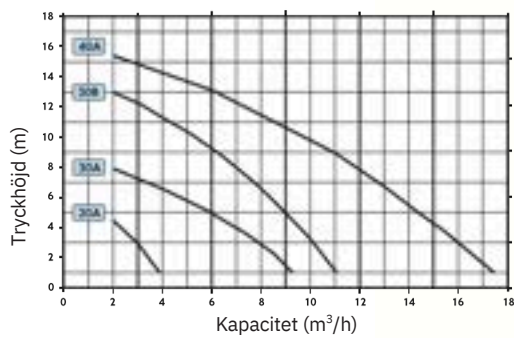
Pumpkurvor Barbera typ AS20–100
