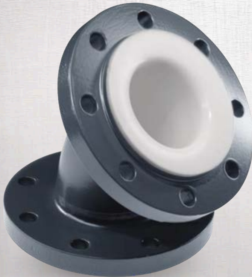
Böj 30°/45°/60°, PTFE-linat, DN15-500
