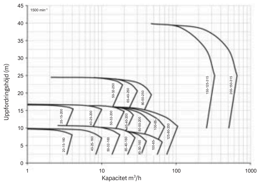
Pumpkurva CP typ MKP 1500 rpm samt 3000 rpm.
